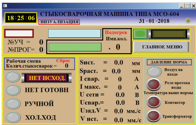
Рис. 1. Фрагмент мультимедийной презентации урока производственного обучения «Настройка режимов сварки на машине контактной сварки МСО-604» (визуализация панели оператора)
