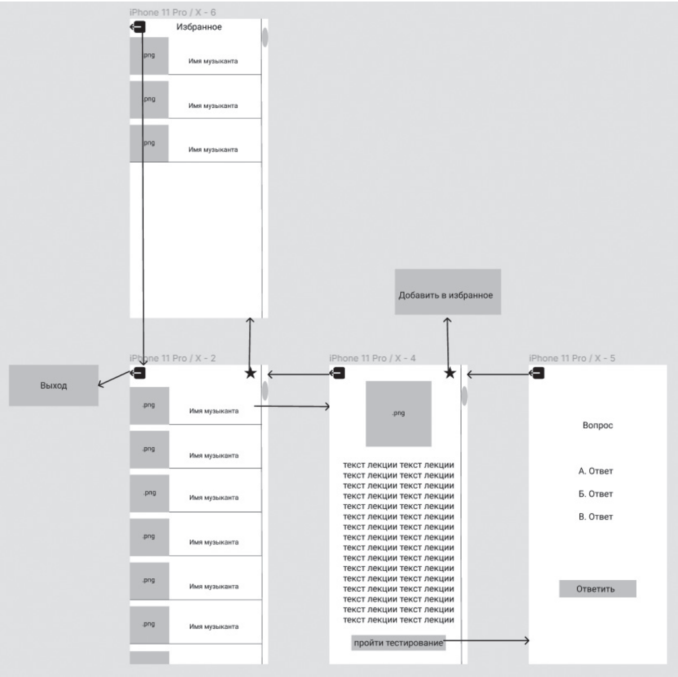
Рис. 12. Прототип приложения «Musical Brain Ring»
