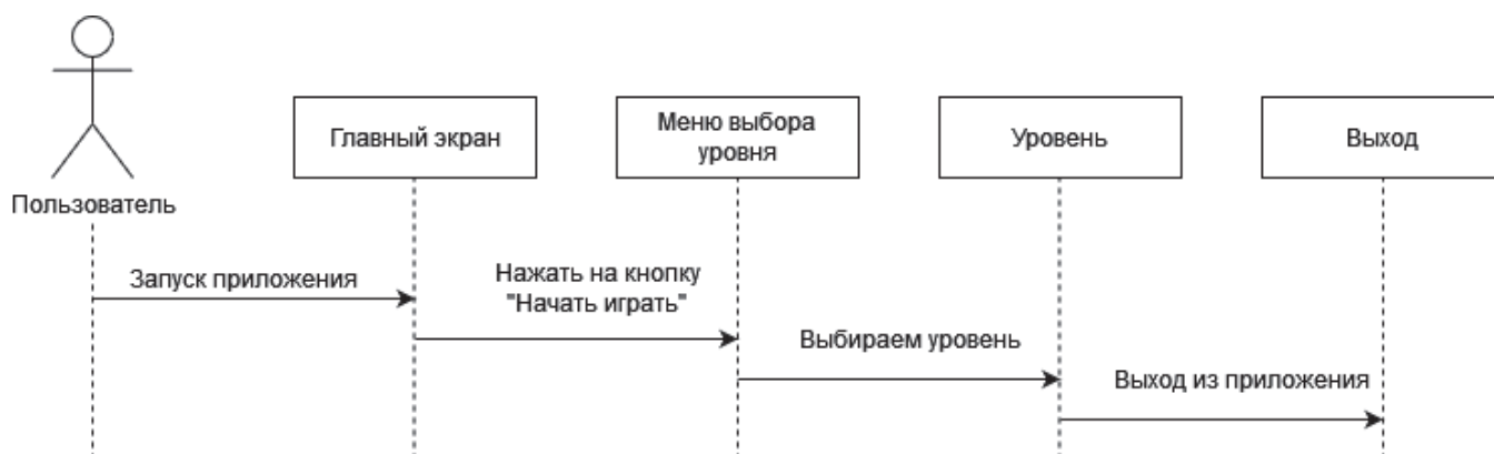
Рис. 6. Диаграмма последовательности
