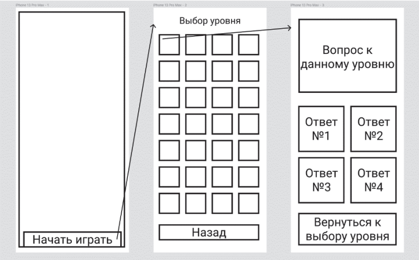
Рис. 1. Прототип приложения «Викторина» а) главное меню б) меню с выбором уровней в) меню уровня
