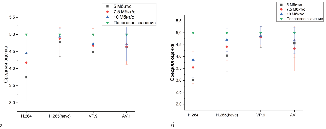
Рис. 3. Общая оценка: а — формата 4К, б — формата 8К
