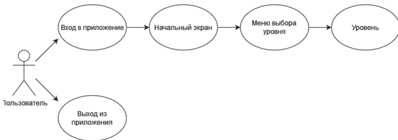
Рис. 5. Диаграмма прецедентов
