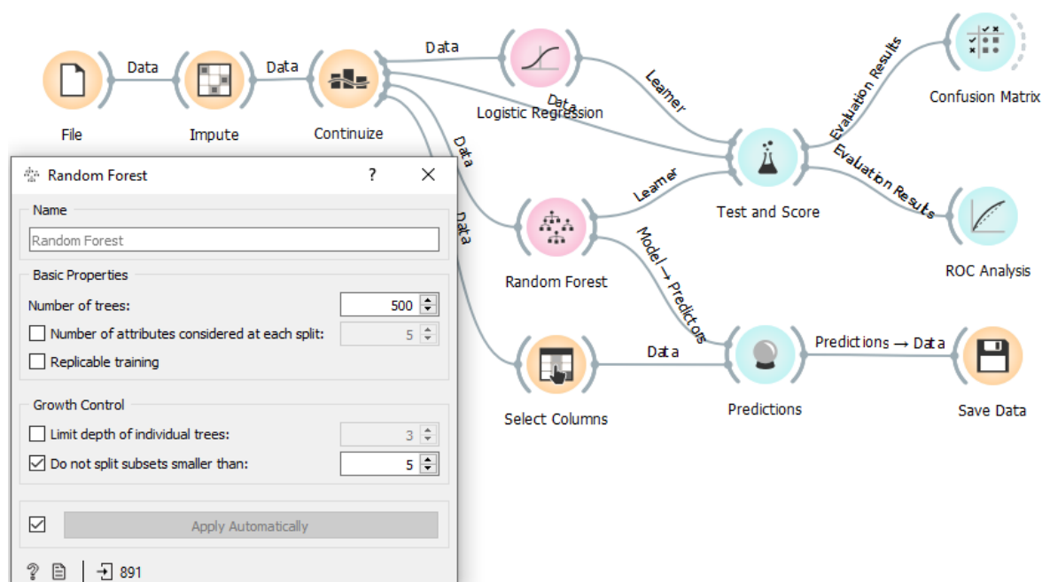
Рис. 2. Решение задачи классификации с помощью Orange3
